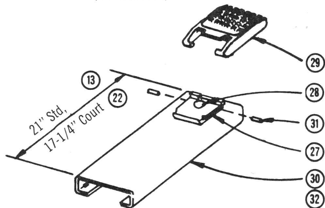
ENSEMBLE DE PATIN ET MANCHON (4 POSITIONS)
